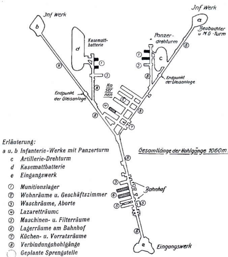
Fig. 4. Gangsystemet i Værkgruppe Berghöhe
